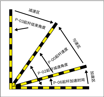
2. 无低速运行区的起杆示意图 (P-25 大于等于 90)
